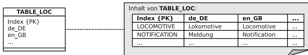
Abbildung 2.4: Neues Datenbankschema – Lokalisierte Tabellennamen
